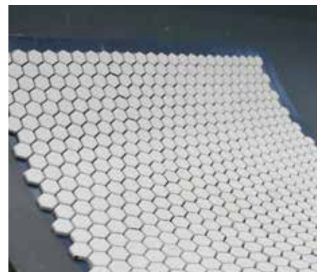
Mit Belzona 1321 verklebte Belzona 9811 Aluminiumoxid-Fliesen
